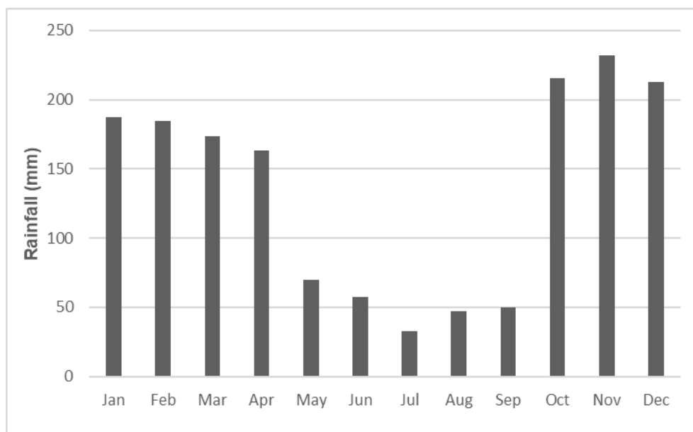
Fig. 3. Mundri Rainfall 2018-2022
