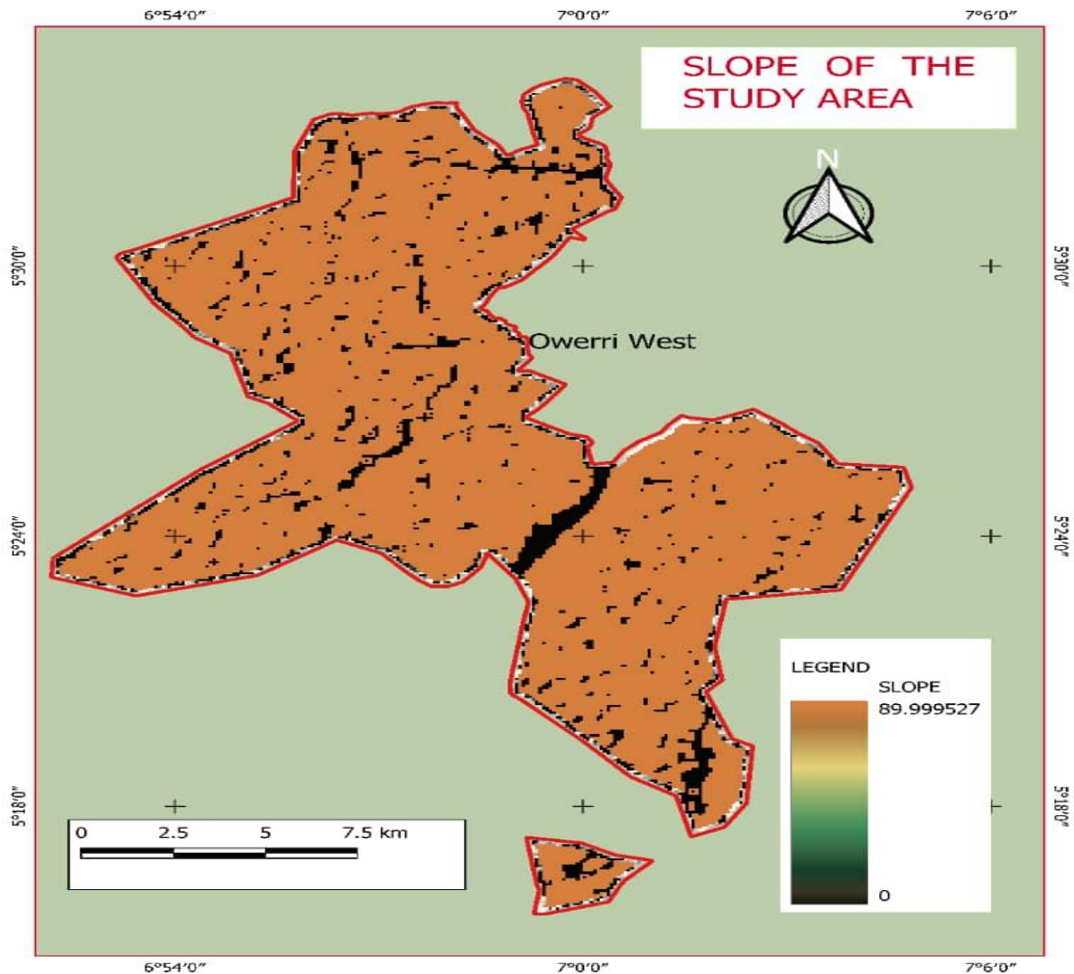
Fig. 7. Slope
