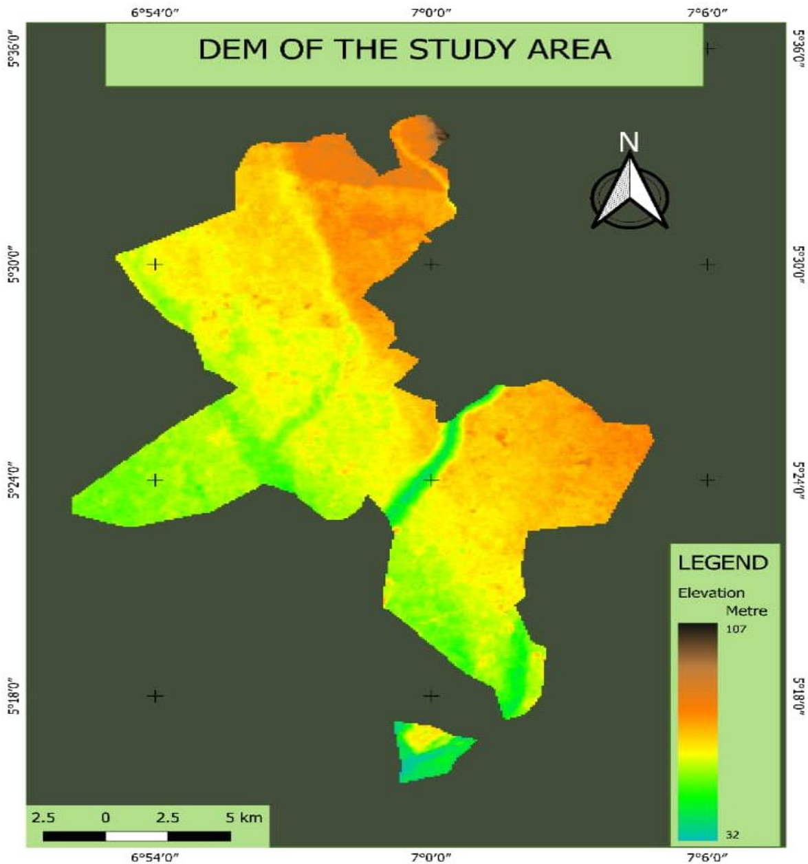
Fig. 6. DEM
