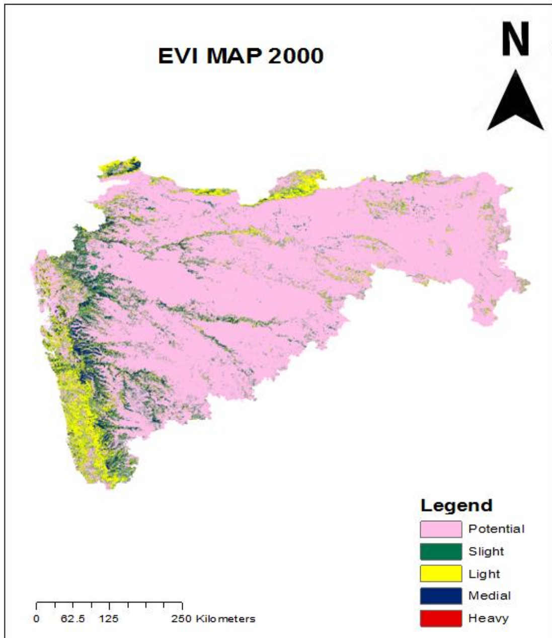
Fig. 3. EVI Map, 2000
